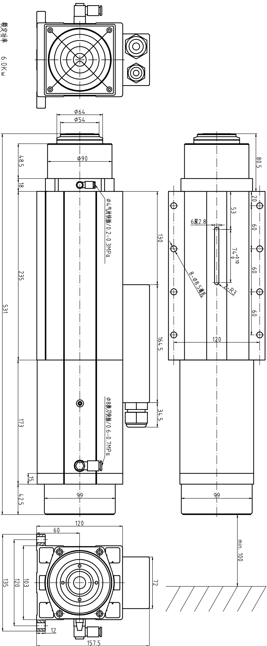
GDL60-30-24Z/6.0 220V外形图
